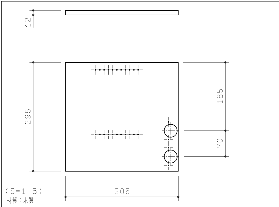
固定扉
