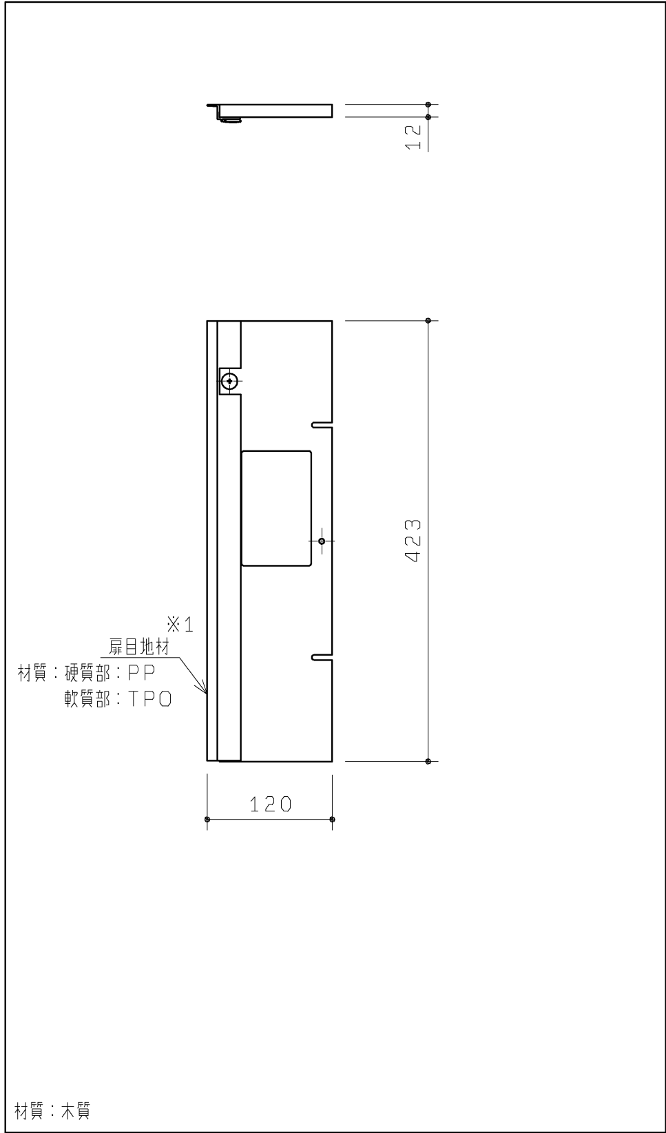
裏扉セット
