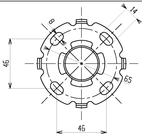
取付座詳細(1:2)
