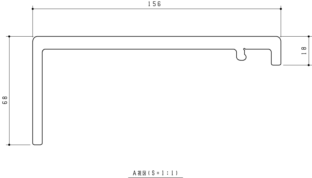
A 視 図 ( S = 1 : 1 )
