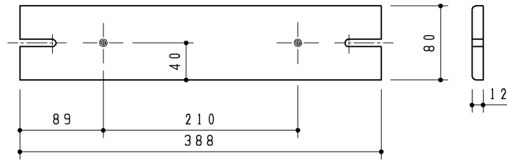
図3 新築用木棧 (同梱部材)
