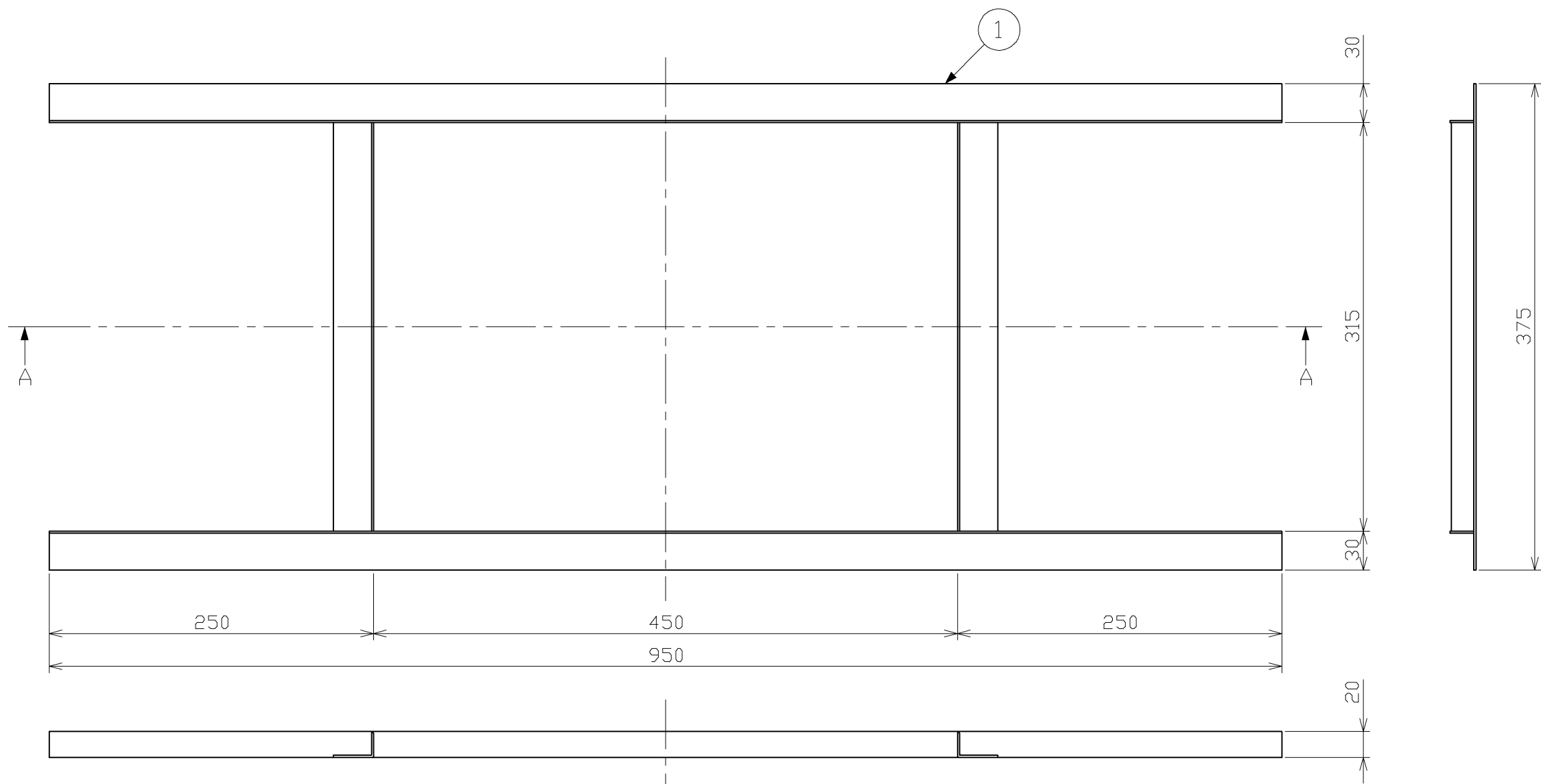
A-A断面図 (1:4)
