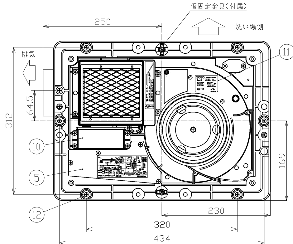
天井取付図 (1:5)
