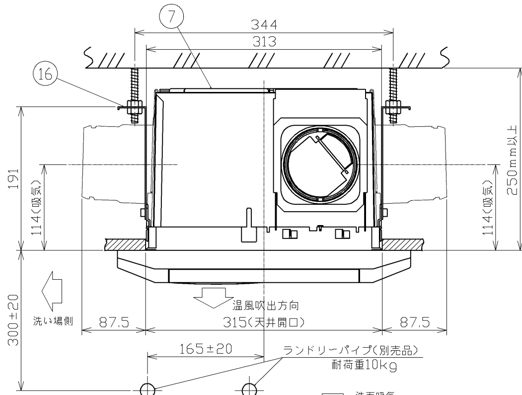
天井取付図 (1:5)
