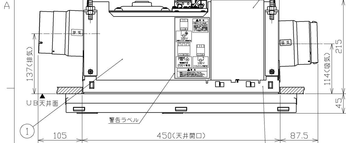
天井取付図 (1:5)
