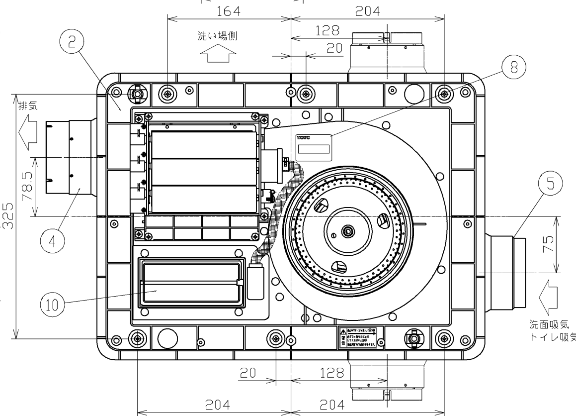
天井取付図 (1:5)
