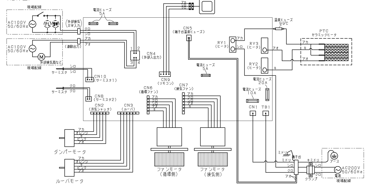
＜結線図＞
