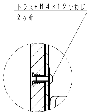
A部詳細 (S=1:2)
