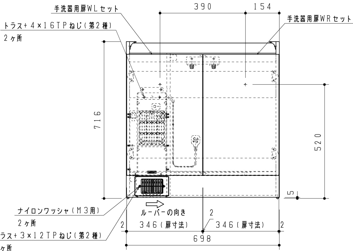
室内暖房ユニット固定詳細
