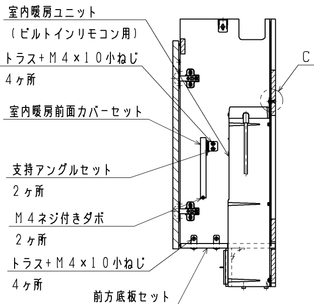
室内暖房ユニット固定詳細
