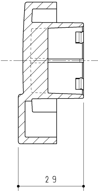
A - A 断面
