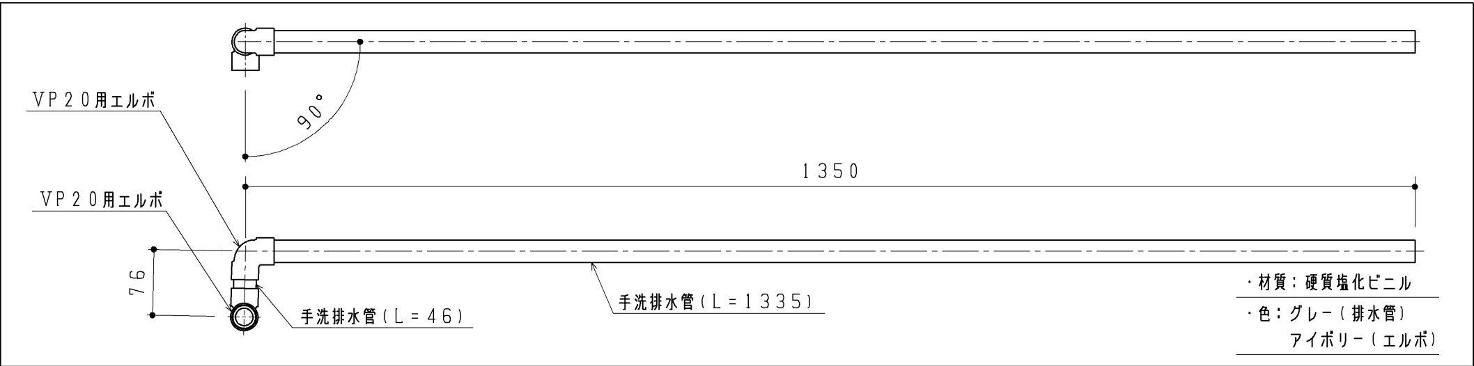
手洗排水横引き管R
