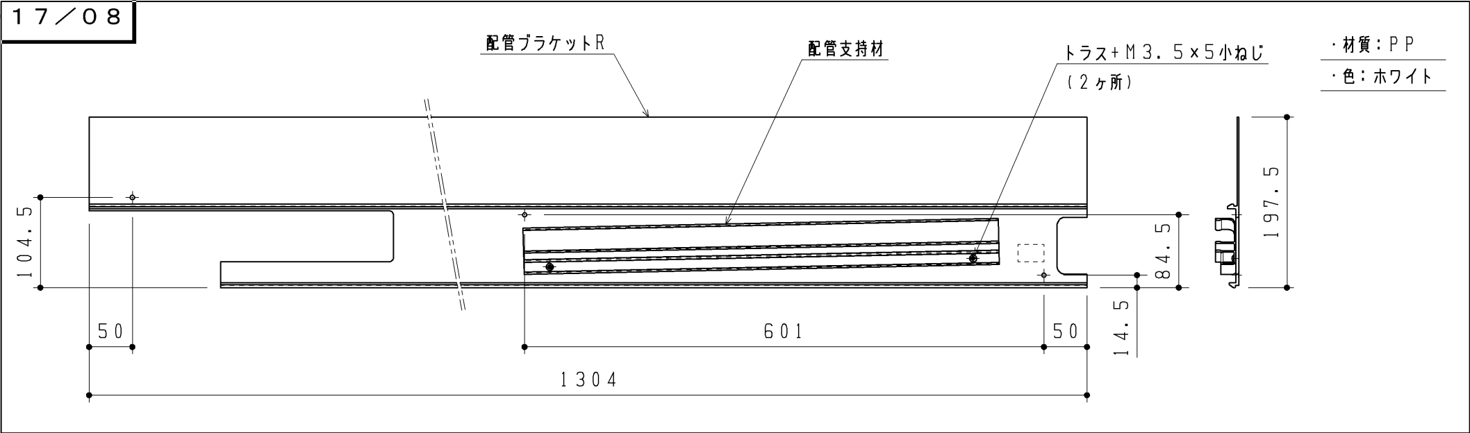
配管ブラケットセットR
