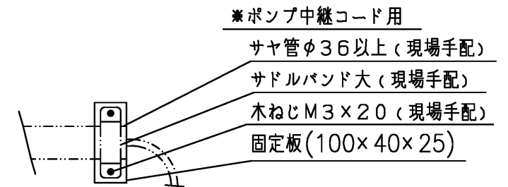
断面 A-A (1:5)
