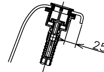
断面B-B(1:5)
