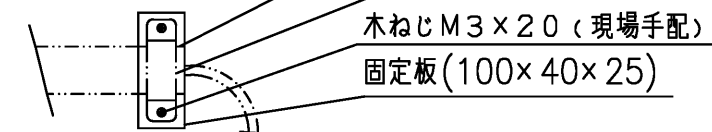
サヤ管固定部詳細図
