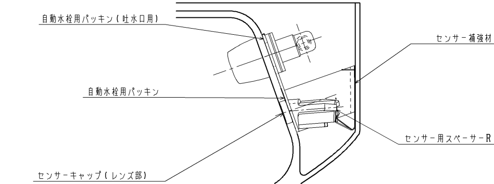
A部断面詳細図(S=1:2)
