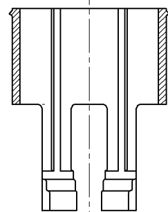
断面C-C
