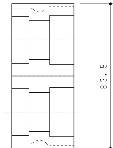
防露カバー（分岐金具部）
