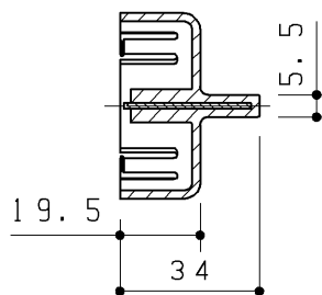
断面A-A
