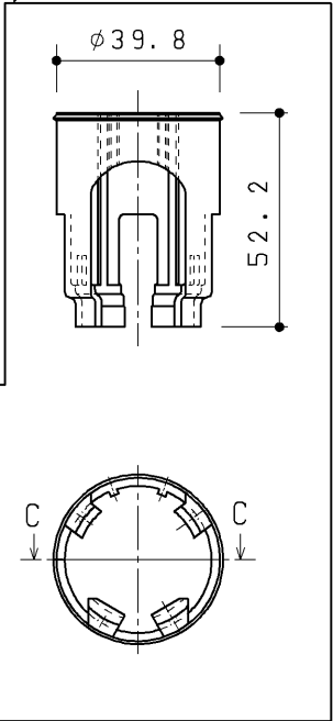
防露カバー(エルボ部、WL用)
