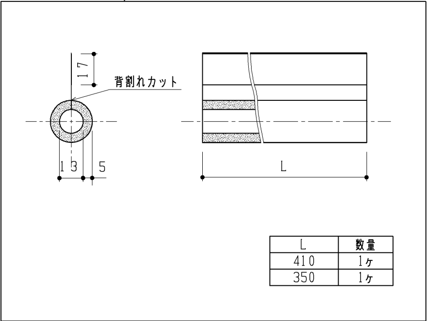
防露カバー(エルボ部、WL用)
