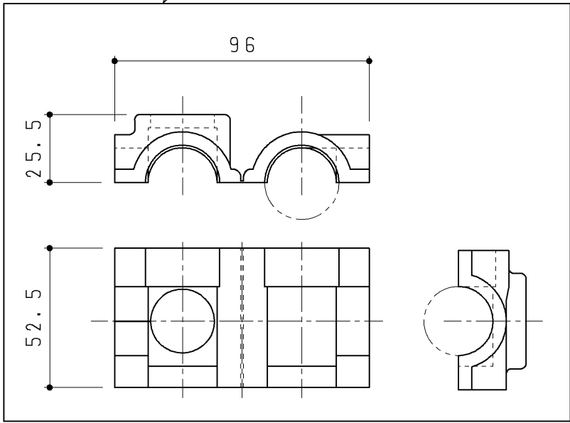
防露カバー(分岐金具部)
