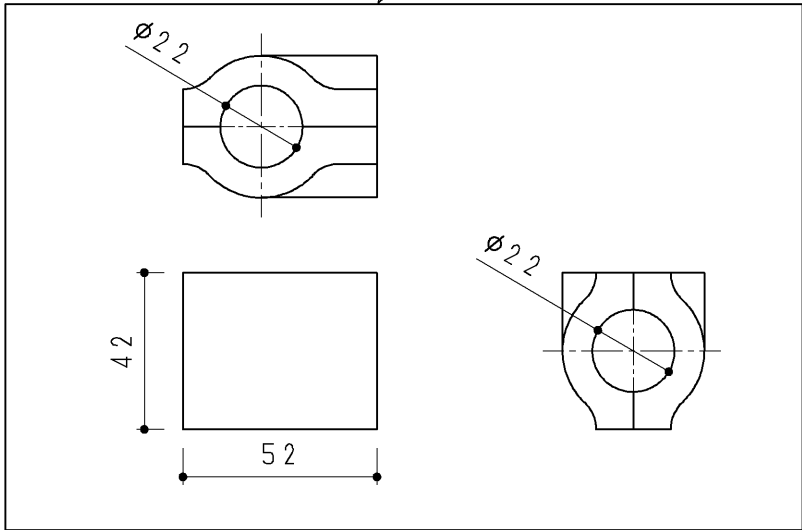
防露カバー(分岐金具部)
