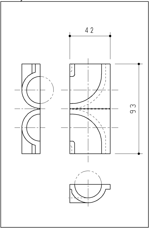
防露カバー(オスメスエルボ用)
