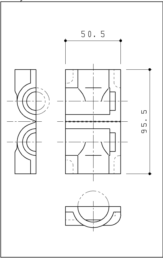
防露カバー(エルボ部、WL用)
