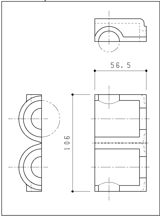
防露カバー(止水栓用)
