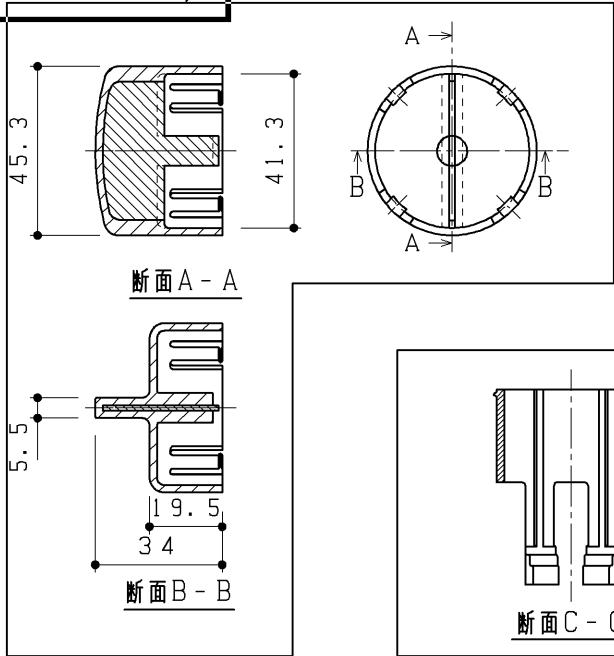
防露カバー(止水栓用)
