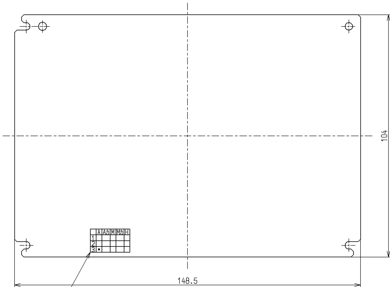
コントローラ基板識別表示
