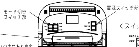
A-A断面図 (下から見た図)
