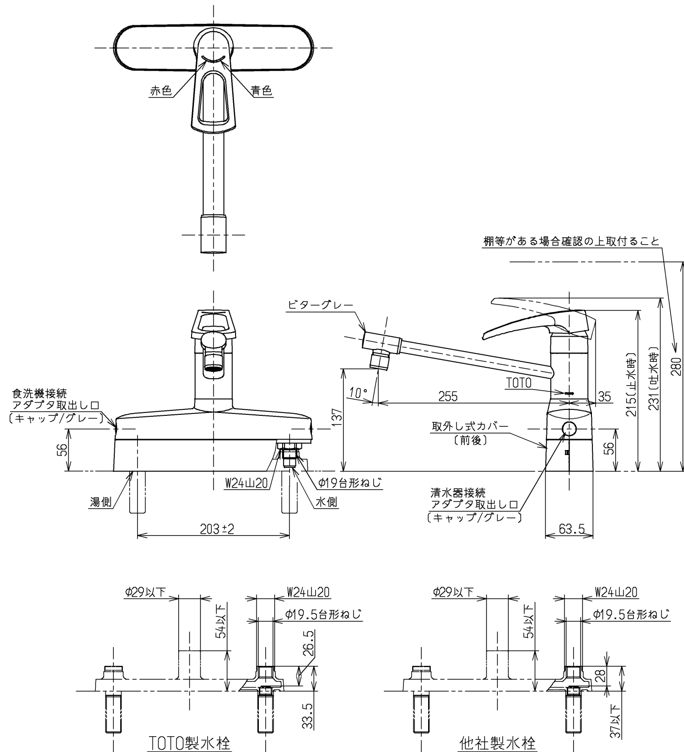
取付可能な水栓の主要寸法
