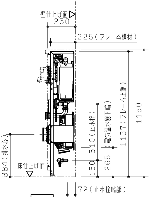
R 視図
