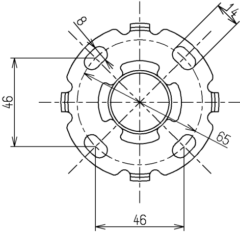
取付座詳細(1:2)
