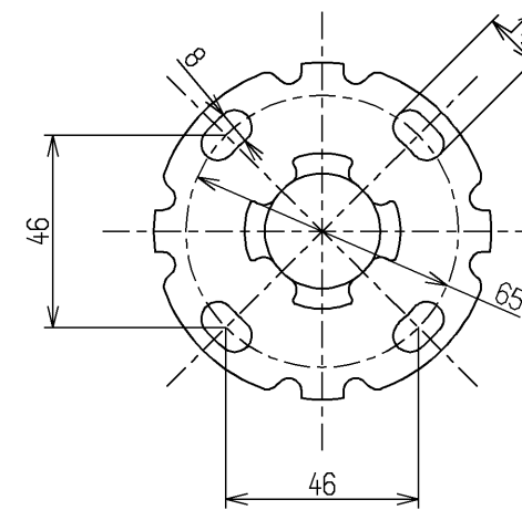
中間部取付座詳細(1:2)
