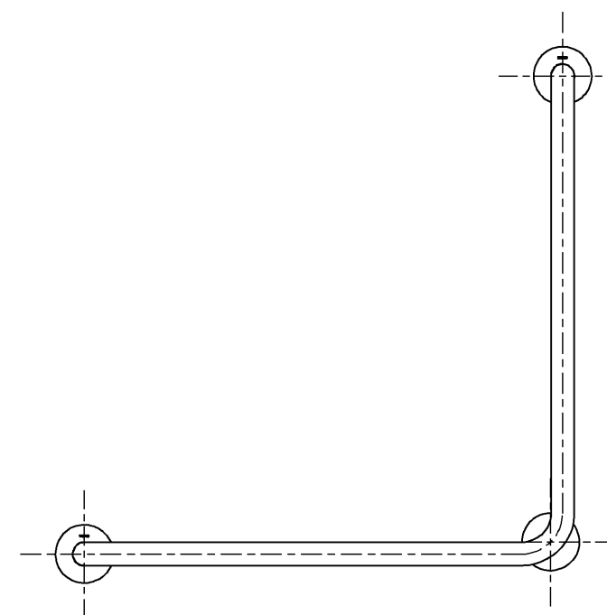
右壁設置の場合 (1:10)
