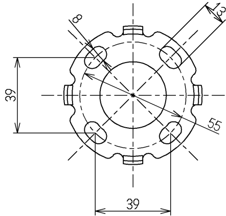
取付座詳細(1:2)
