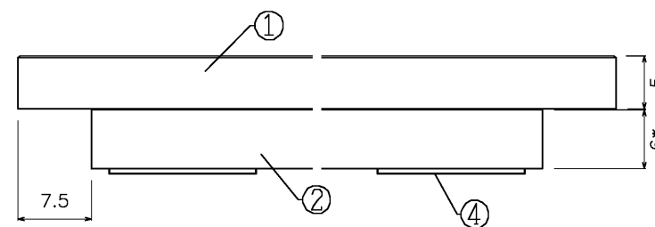
B-B断面図
