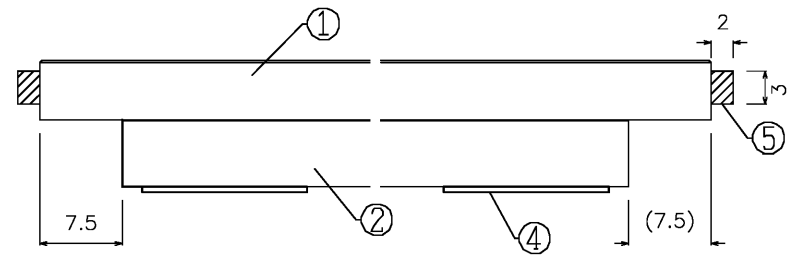
A-A断面図
