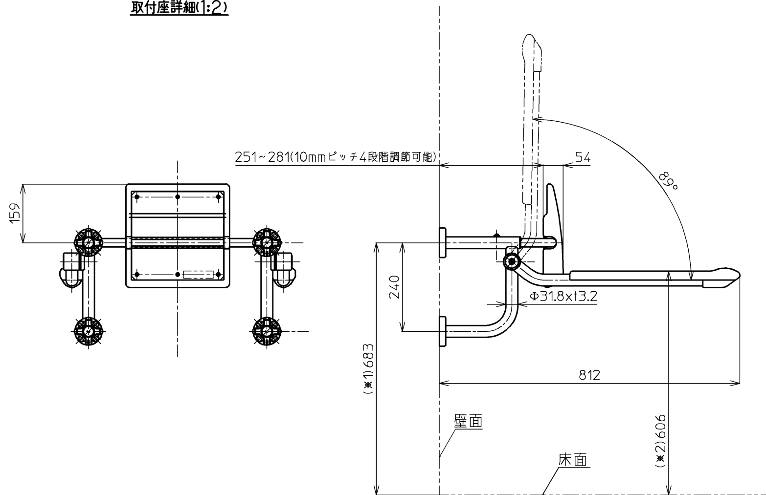
取付座詳細(1:2)
