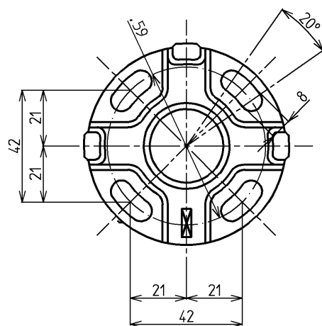
取付座詳細(1:2)
