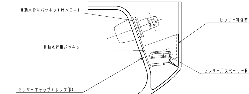
A部断面詳細図(S=1:2)
