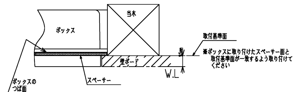
壁厚み別ボックス取り付け位置詳細図
