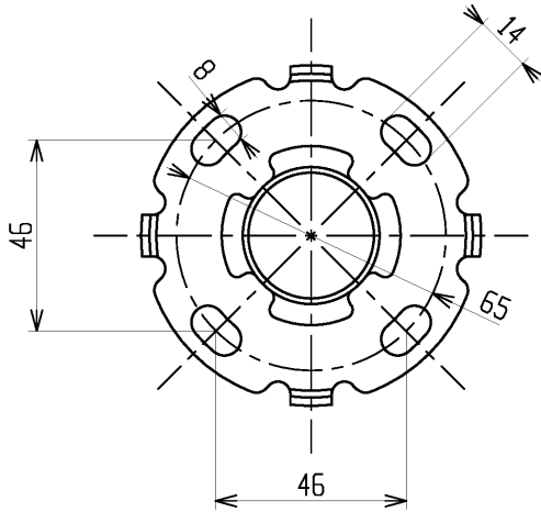
取付座詳細(1:2)
