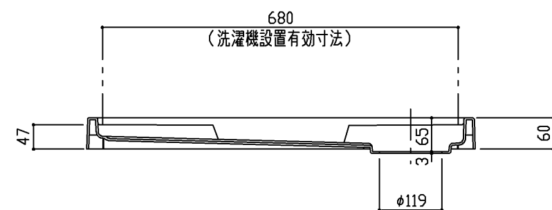
断面A-A
