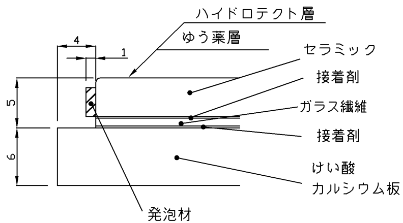
A, C部(断面図)拡大図
