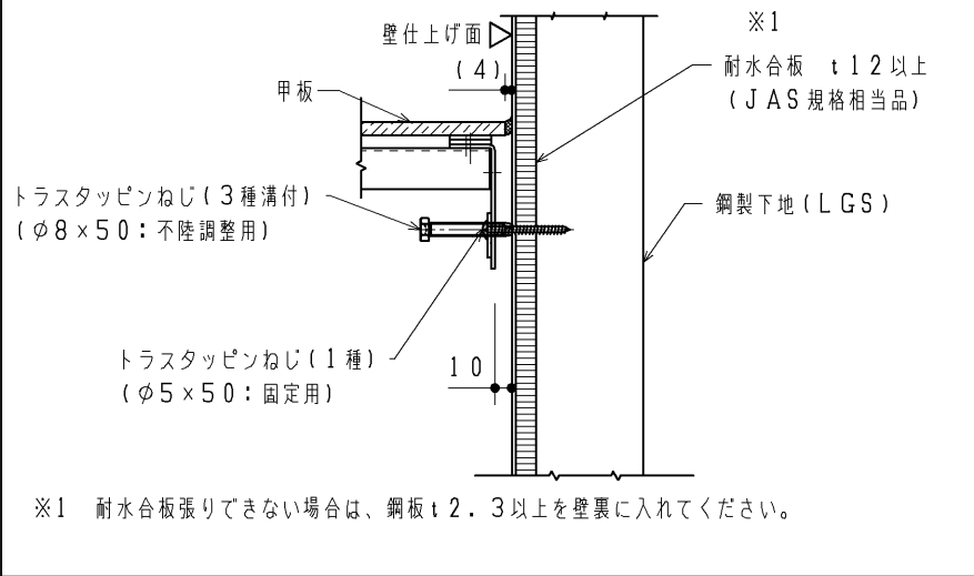
【甲板部納まり詳細図 (S=1:5)】
