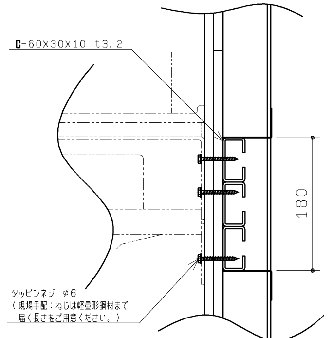
※3補強木の代わりに軽量形鋼材 C-60x30x10 t3.2 を入れた場合のB部詳細図 1/5
