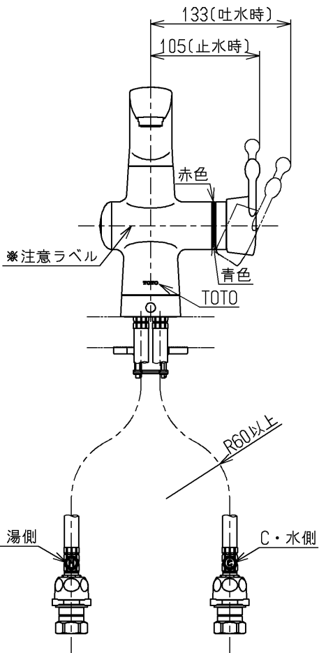
上面施工 ウォーターハンマー低減機構内蔵
