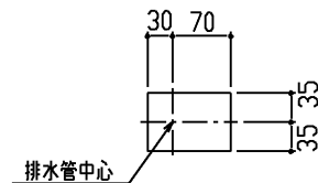
排水穴あけ要領 (1:10)
