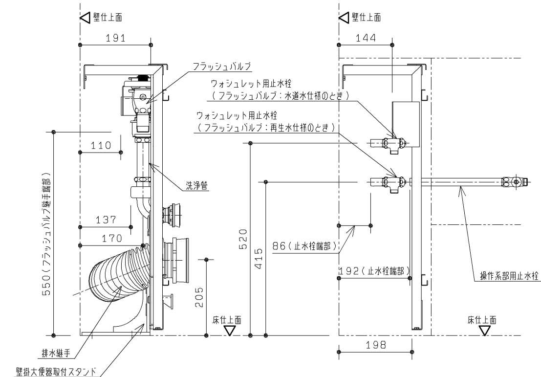
R 視図
