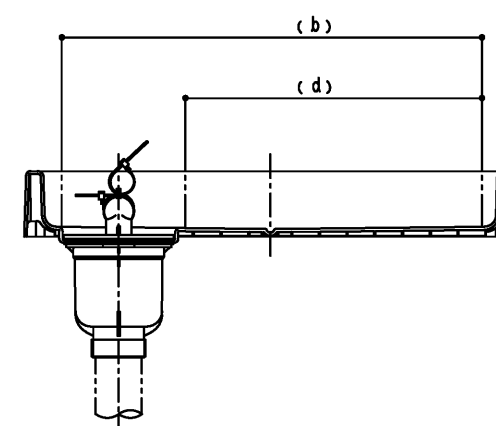
断面B-B
