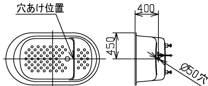
追焚用穴あけ可能位置(1:40)
