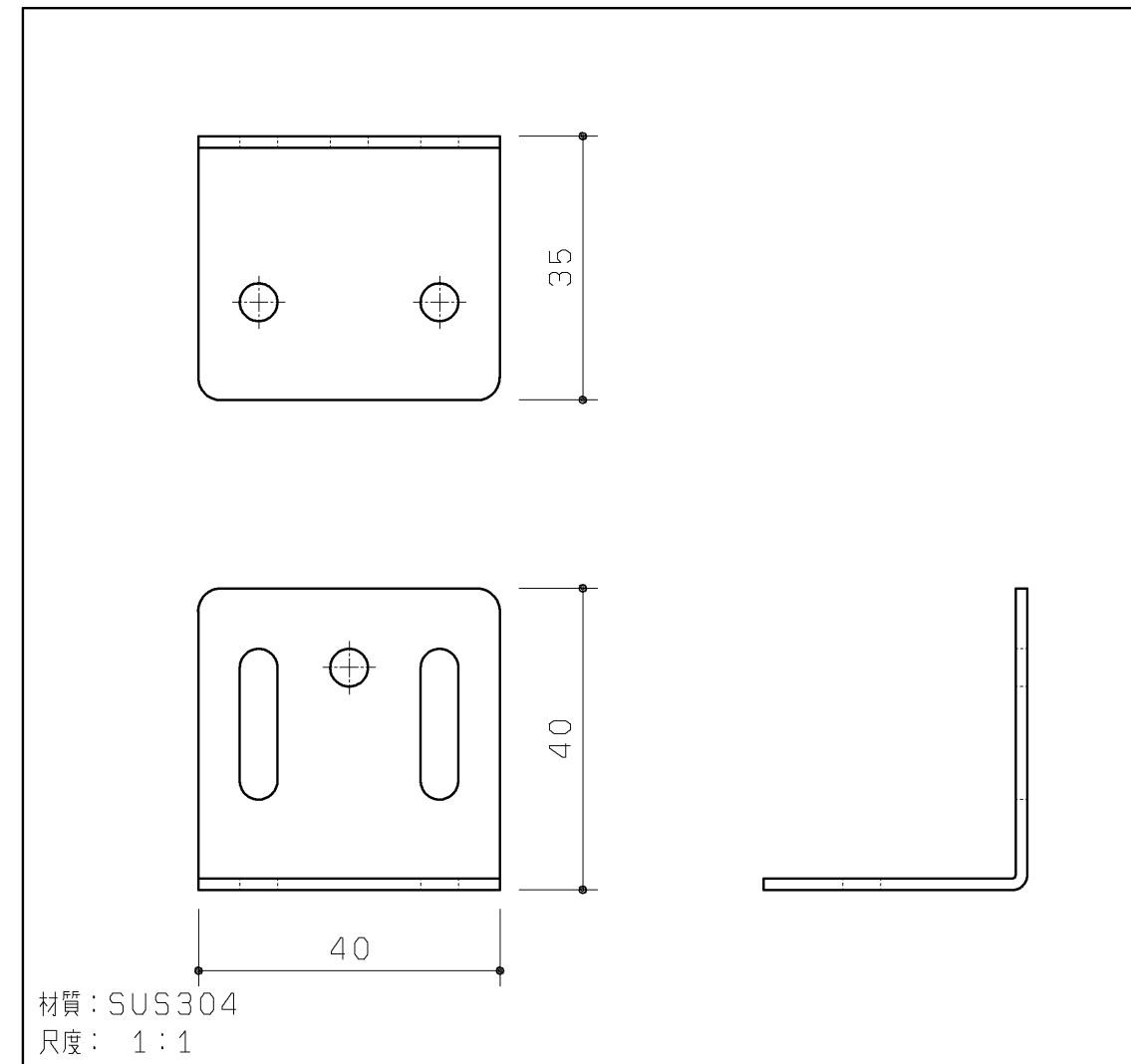
アングル材 ( 3ヶ )
