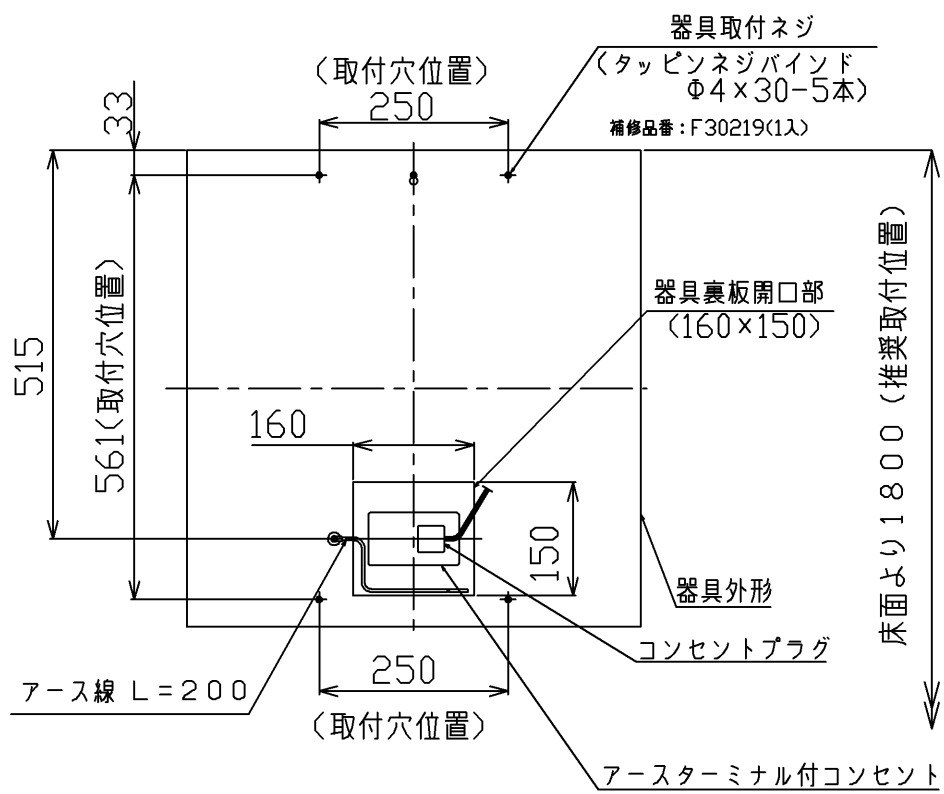
器具取付要領 (S=1/10)
