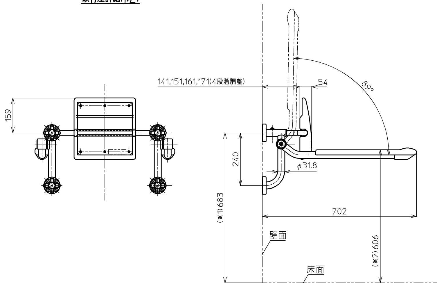
取付座詳細(1:2)
