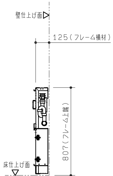
Q 視図
