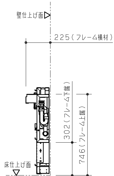
P 視図
