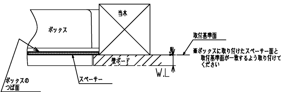
壁厚み別ボックス取り付け位置詳細図
