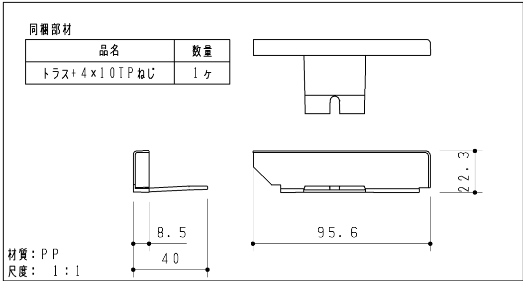
カウンターキャップセット
