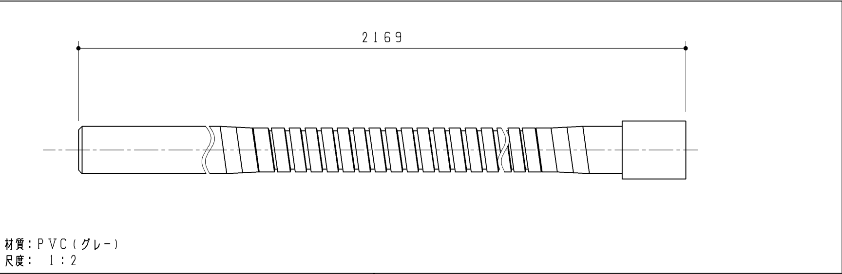
手洗排水ホースセット
