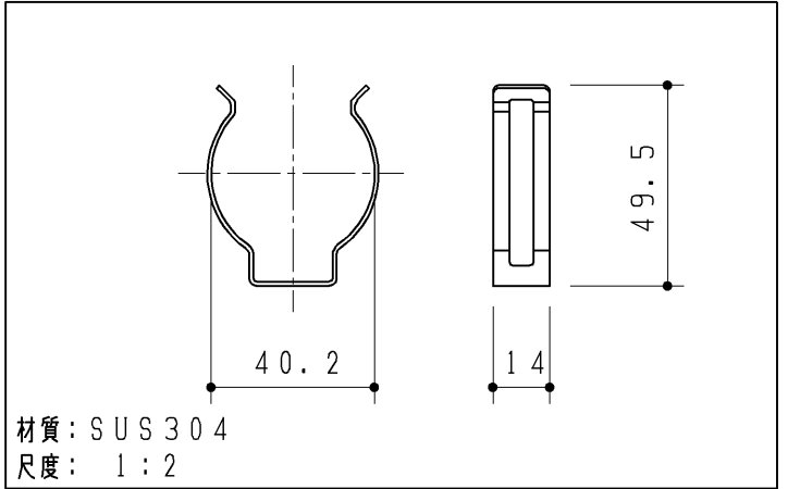
クイックファスナー
