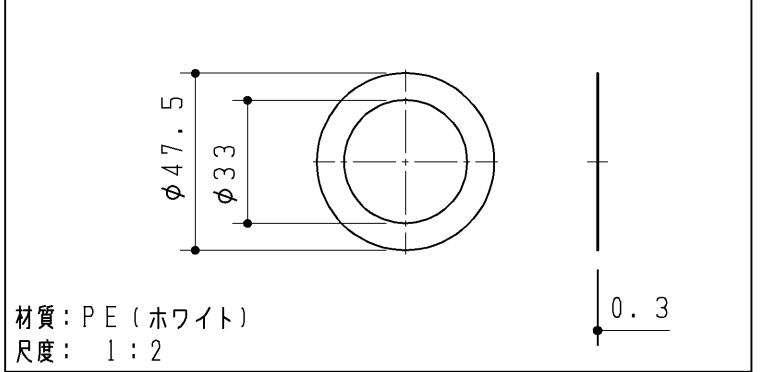
手洗器排水用スリップワッシャ
