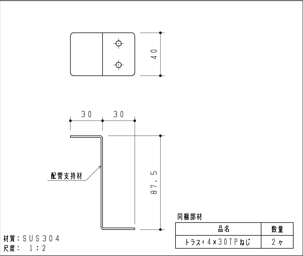
配管支持材セット
