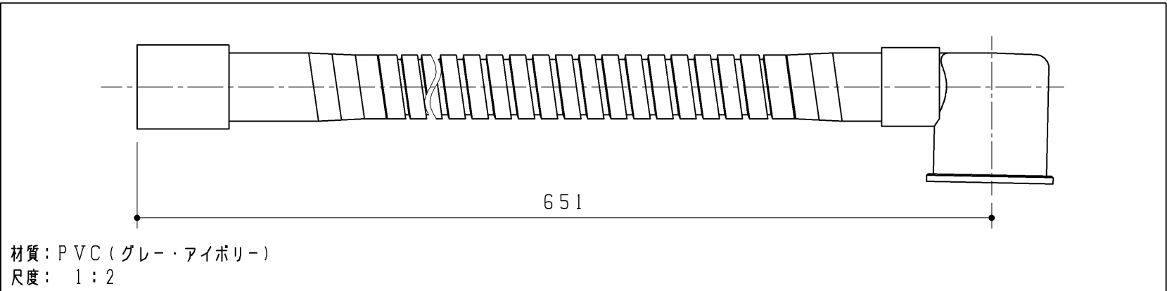
トラップ排水管セット
