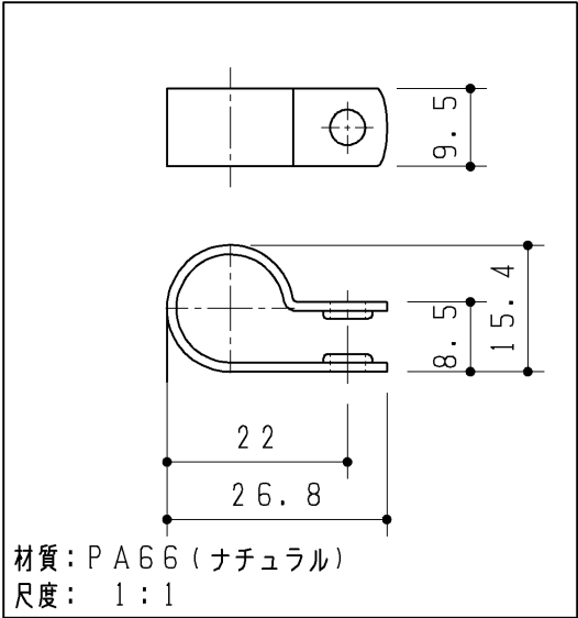
ホースクランプ (3ヶ)
