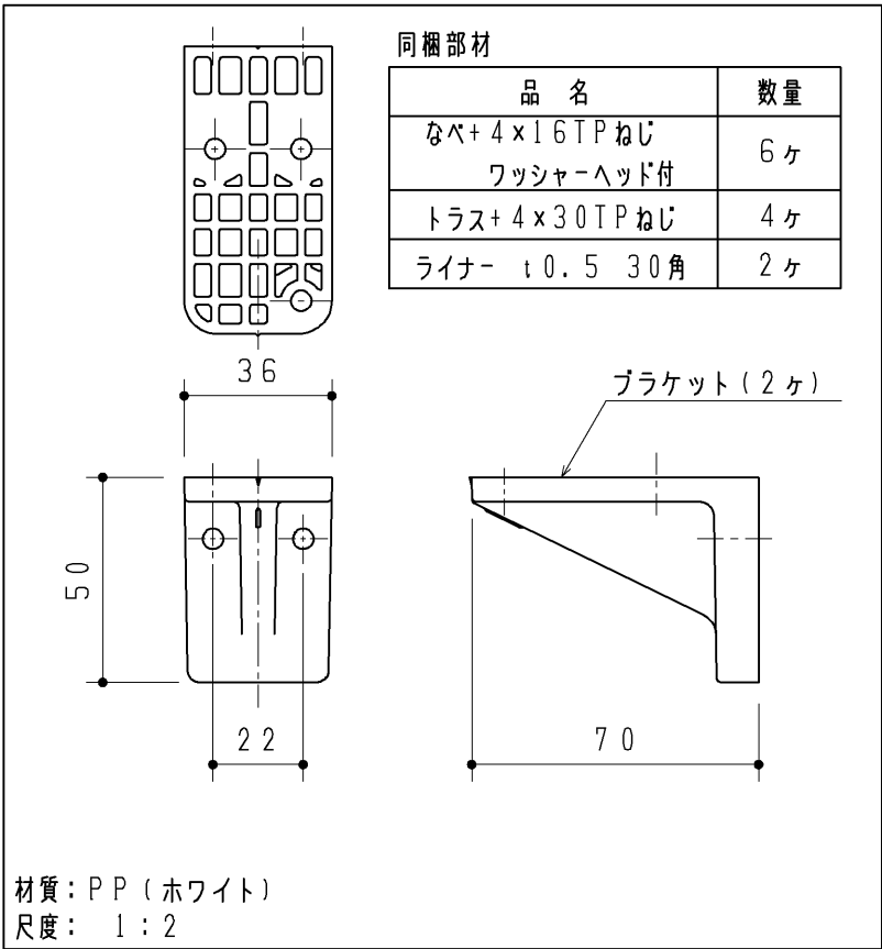
ブラケットセット
