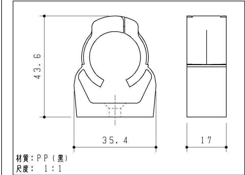
配管固定材 (3ヶ)
