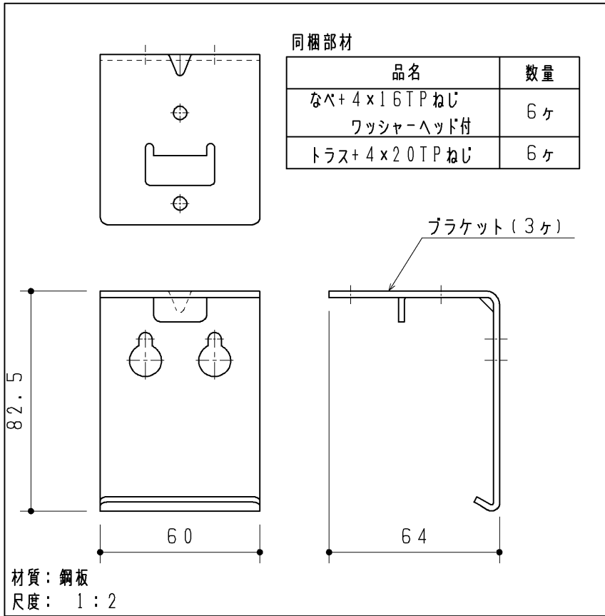
下段ブラケットセット
