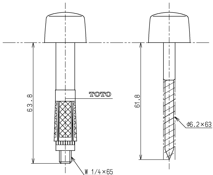
AYボルトを使用の場合
