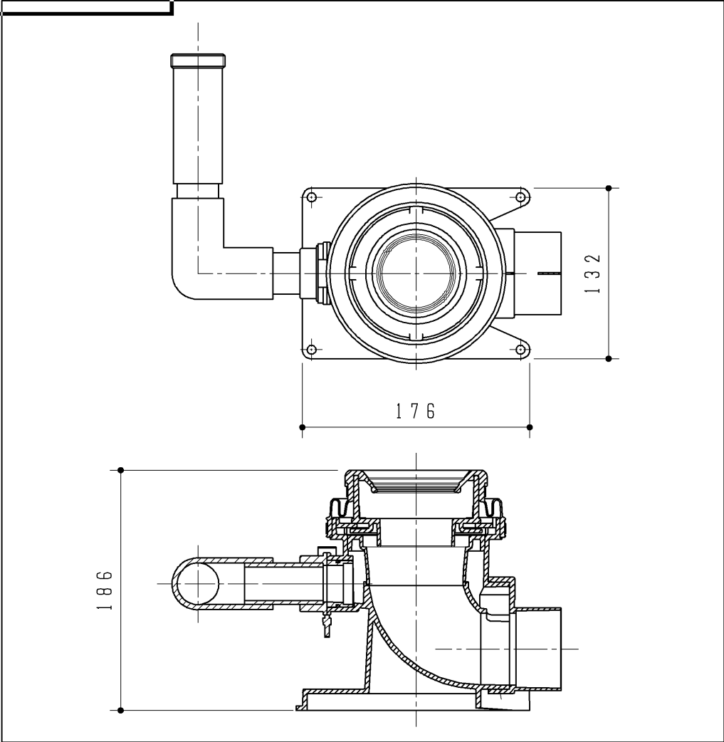
手洗排水管（間口調整用）
