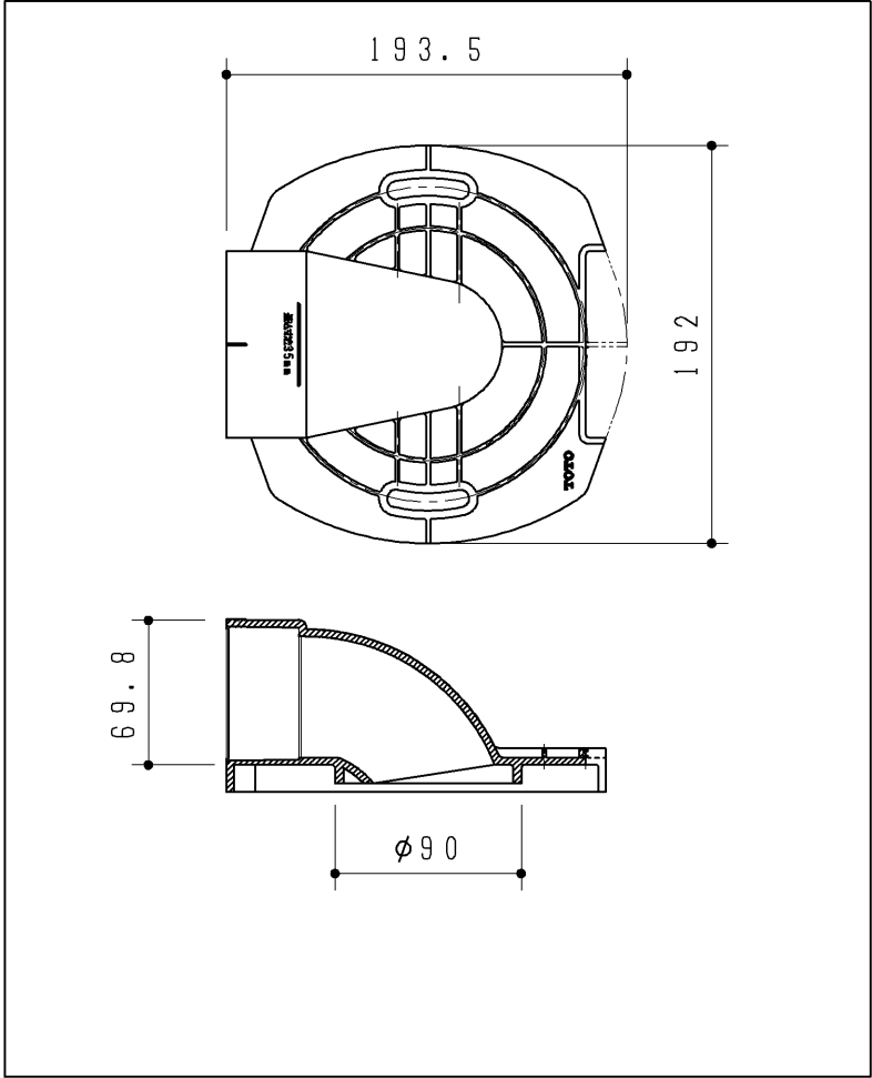
固定片（前）
