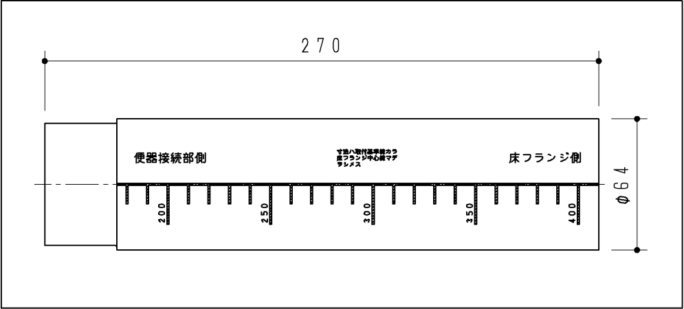
手洗排水縦管
