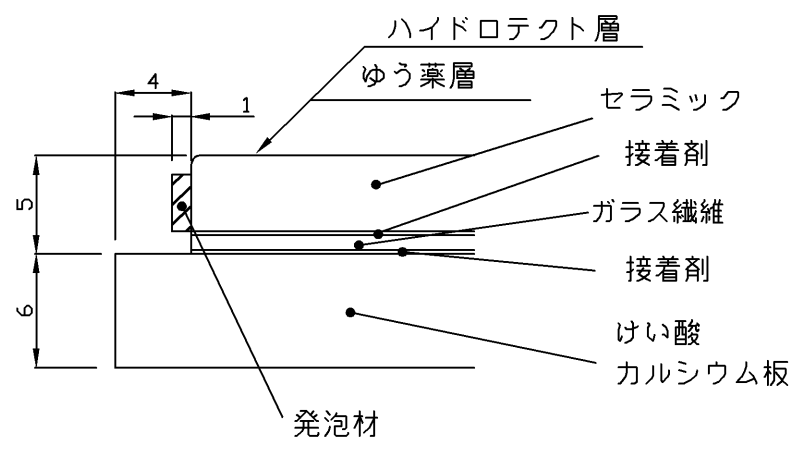
A, C部 (断面図) 拡大図
