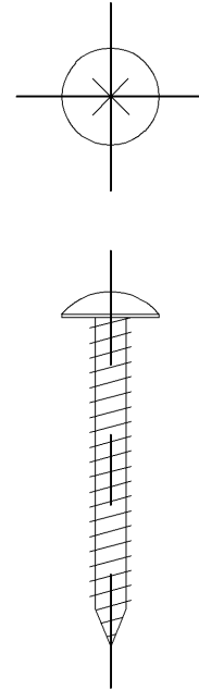
JIS B1122 十字穴付きタッピンねじ トラス4種5×40 (市販品でも可)
